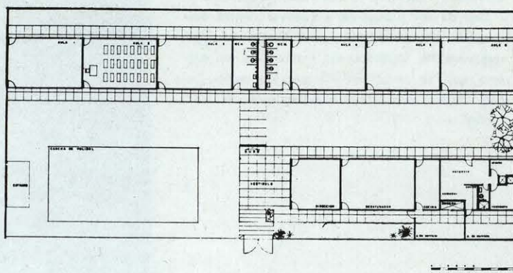
Planta y alzado principal de la escuela primaria mixta para 300 alumnos, en Pachuca.
