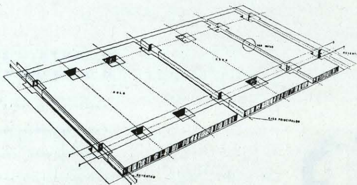
Planta de cimiento.
