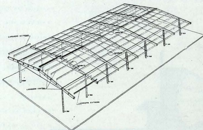
Estructura.
