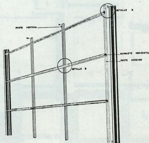
Estructura. Módulo de cerramiento.
