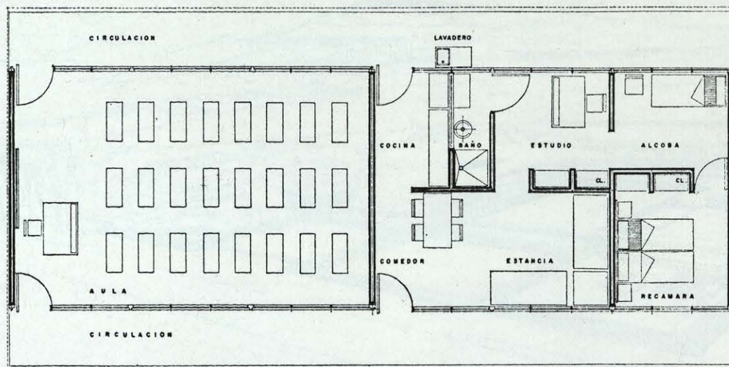
Planta aula-casa.
